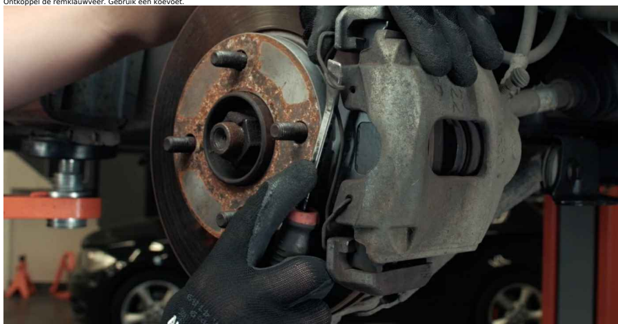
11 Verwijder de remklauw.
