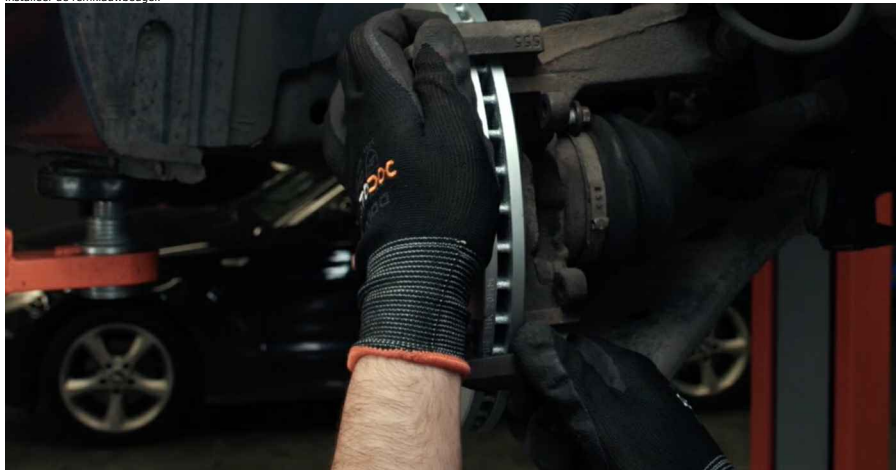
21 Span de remklauwbeugel aan. Gebruik een dopsleutel Nr.13. Gebruik een momentsleutel. Draai deze vast tot een koppel van 70 Nm.
