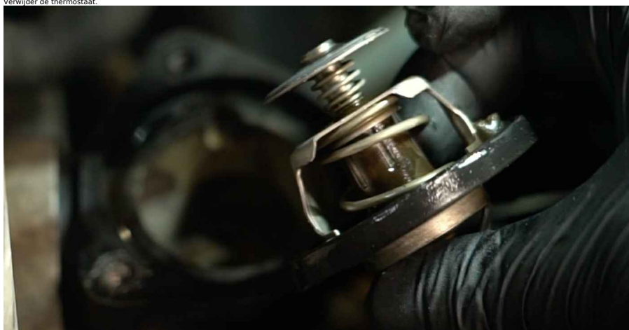
16 Reinig de montageplek van de kap van de thermostaatbehuizing. Gebruik een universele reinigingspray.
