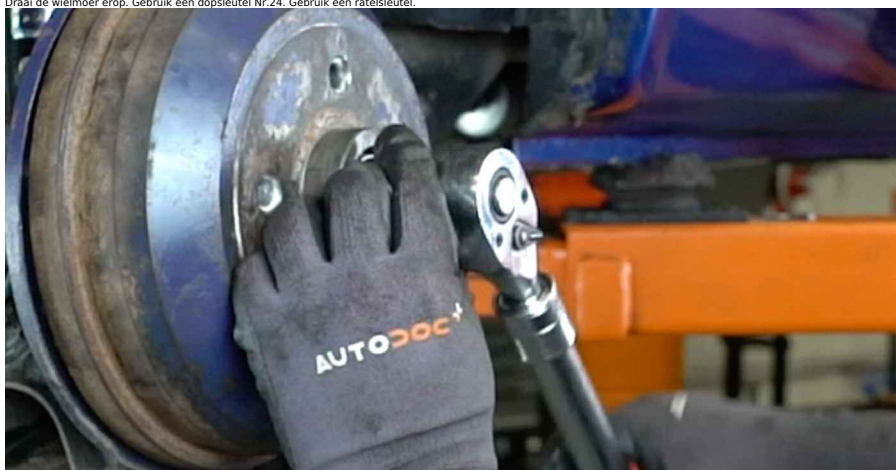
47 Draai de wielbouten vast. Gebruik de kracht dopsleutel #17.
