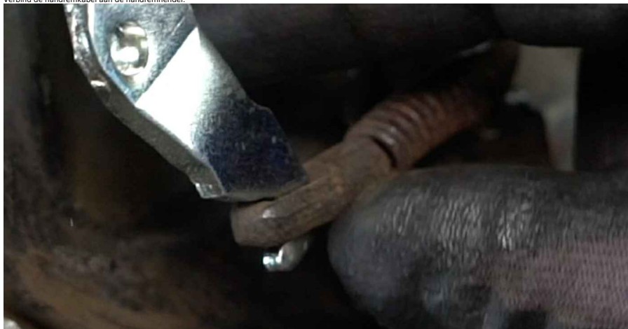
24 Installeer een nieuwe linker remschoen.
