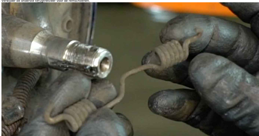
20 Ontkoppel de handremkabel.
