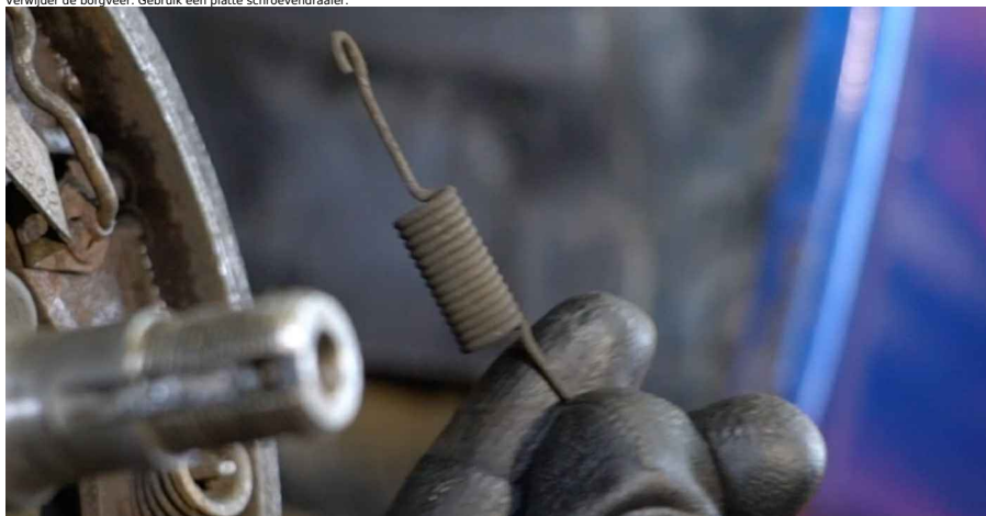
16 Verwijder de houders van de remschoenen. Maak gebruik van een borgveertang voor het spannen van remschoen-borgveren.
