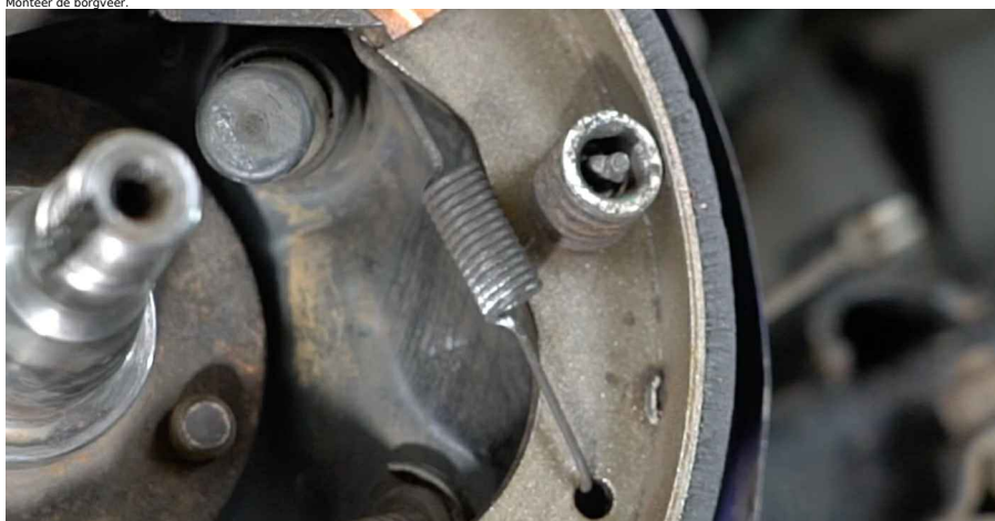
40 Monteer de bovenste terugtrekveer. Maak gebruik van de langbektang.
