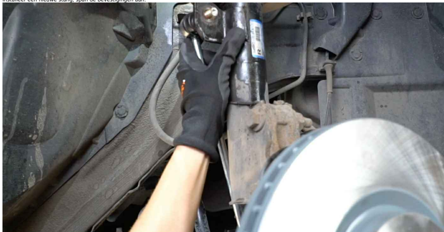
12 Draai het bevestigingsstuk dat de koppelstang en de stabilisatorstang met elkaar verbindt vast. Gebruik een combinatie steeksleutel Nr.19 Gebruik een dopsleutel Nr.19. Gebruik een momentsleutel. Draai deze vast tot een koppel van 65 Nm.
